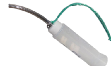
初乳・薬液用ボトル 400ml ホース付(13cm×12φ) 寸法:36×6.5×6.5cm 重量:72g
