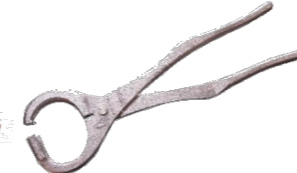
モーリング専用ハンドパンチ 先端にモーリングを装着して牛に通します。
